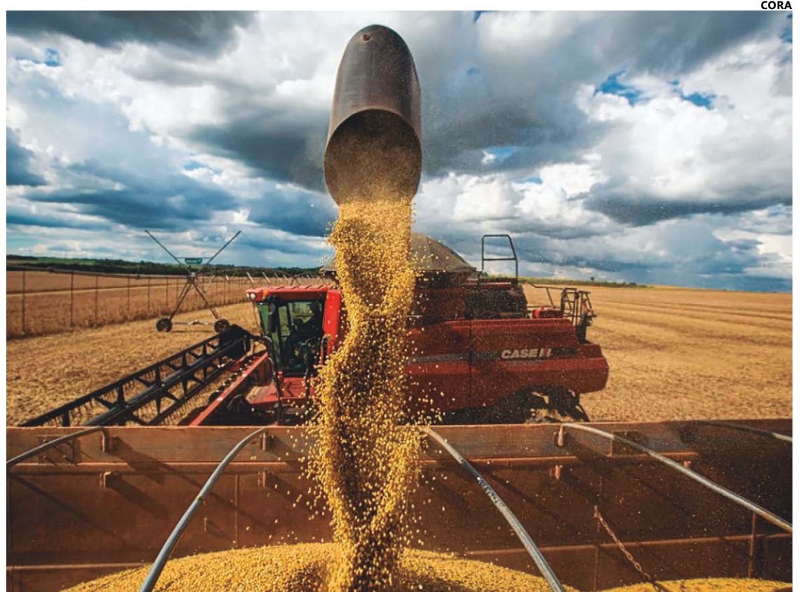
Dados do Agro mostra que em 2022 o Valor Bruto da Produção Agropecuária de Goiás foi o 5º maior do país
